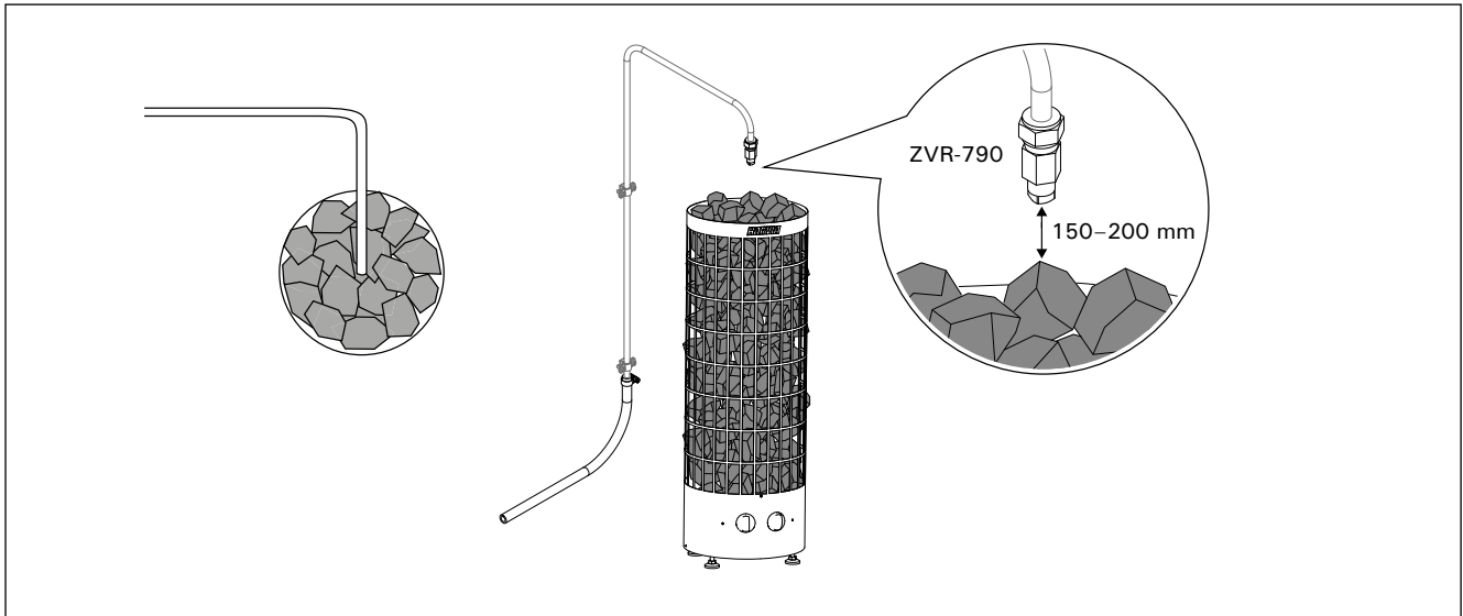
Figure 4. Installation of nozzle Abbildung 4. Montage der Düse
